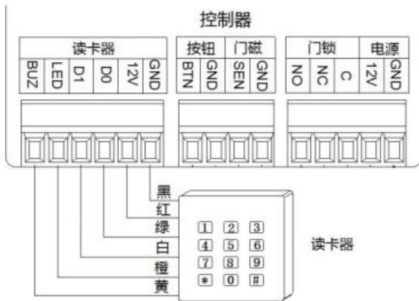
图 4：读卡器接线示意图
