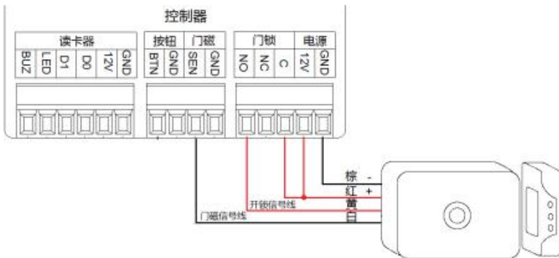
图 7：电控锁接线示意图
