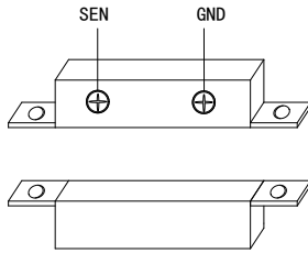
门磁实物图
