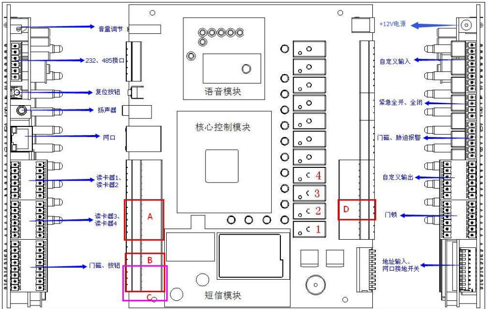
图 1: DW-6802B 控制板结构图
