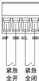
图 7: 紧急全开全闭示意图
