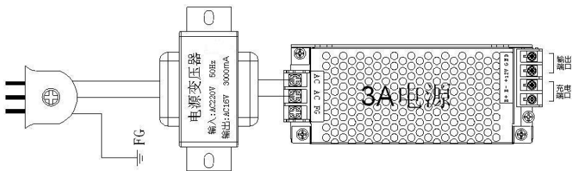
图10: 3A电源连线图
