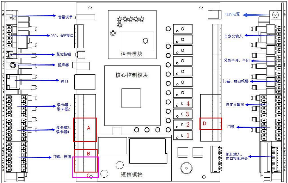
图 1：门控制板结构图
